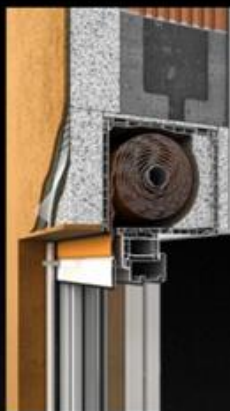
roleta zabudowana całkowicie
