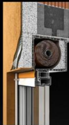
roleta zabudowana częściowo
